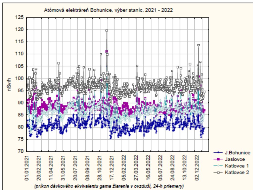
Obr. 1 Slovenské elektrárne, grafický priebeh 24-h priemerov, 2021 - 2022 elektrárne Bohunice
